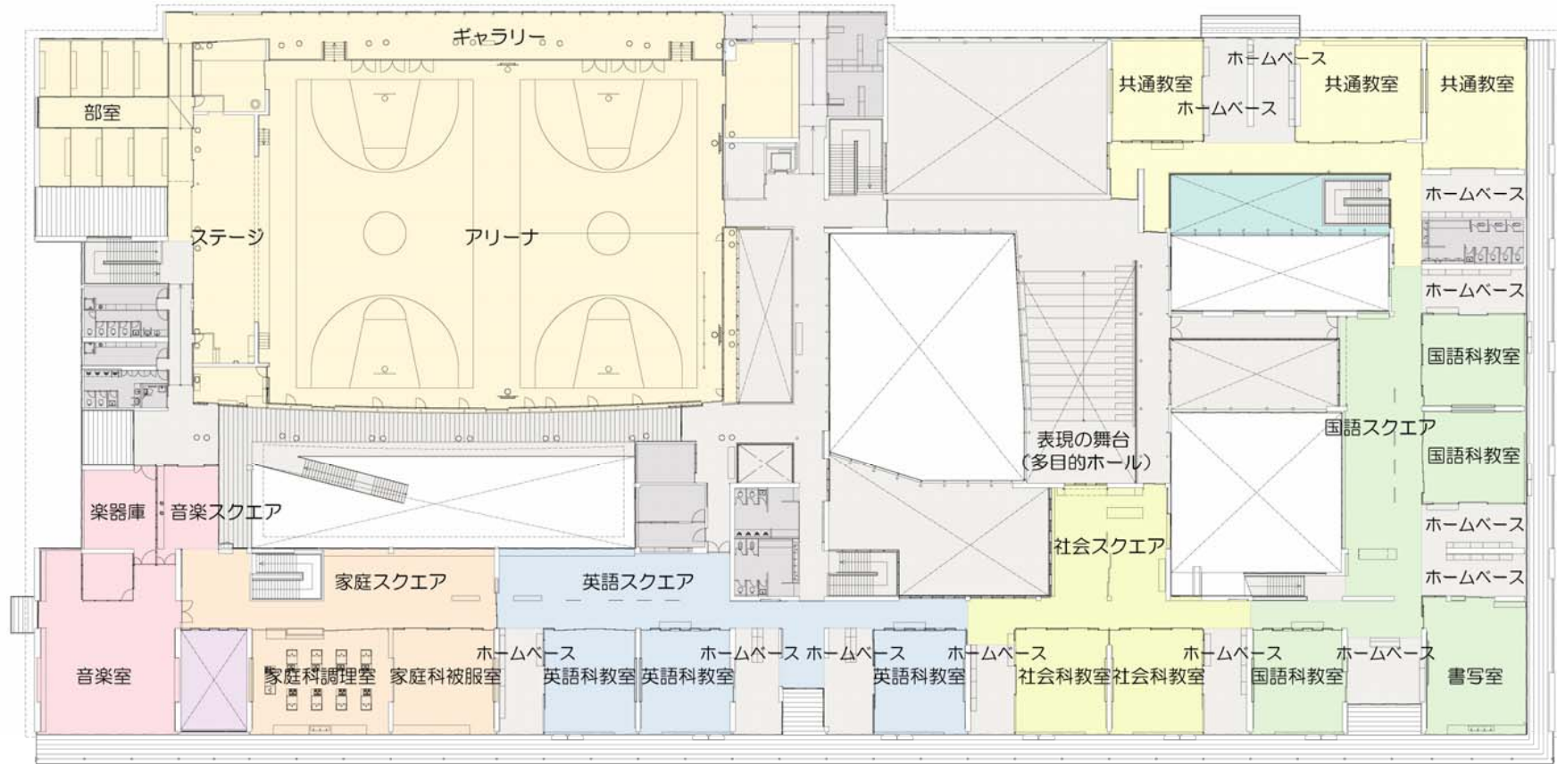
2階平面図
